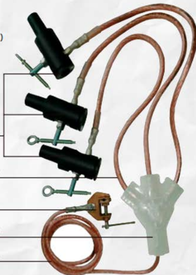
Mordaza de contacto para conexión de conectores codo 15kV 200A.
