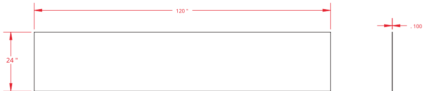
HOJA DE SILICONA PARTE #: E / SS-24 No de DWG: 330 - 00-01
