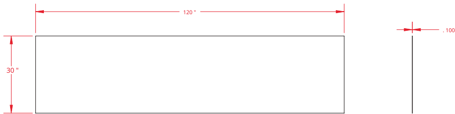
HOJA DE SILICONA PARTE #: E / SS-30 No de DWG: 330 - 00-02
